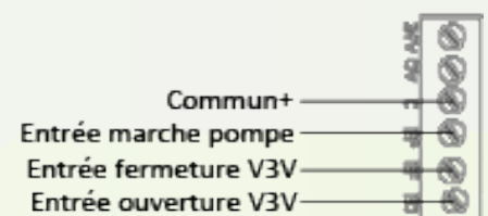
3.1. Commande 24Vdc extérieur
