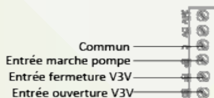
3.1. Commande 24Vac extérieur
